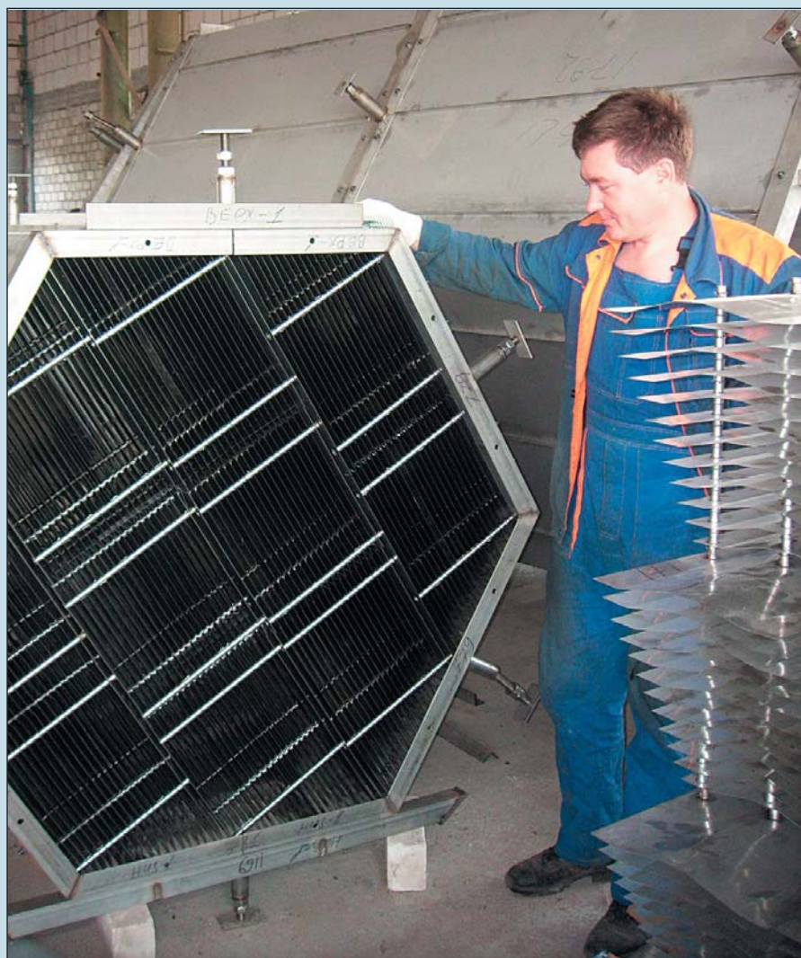
Пробная сборка внутренних устройств горизонтального цилиндрического отстойника
